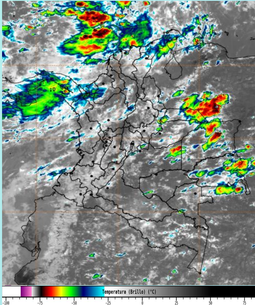
Imagen GOES 19 East Canal Infrarrojo, 11 de octubre de 2025 - Hora 11:50 HLC. IDEAM – GOES 19
