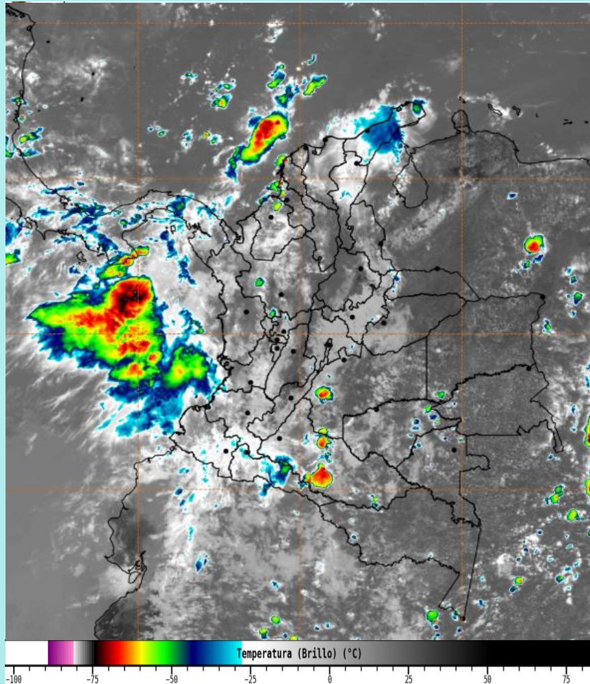
Imagen GOES 19 East Canal Infrarrojo, 1 de octubre de 2025 - Hora 12:10 HLC. IDEAM – GOES 19
