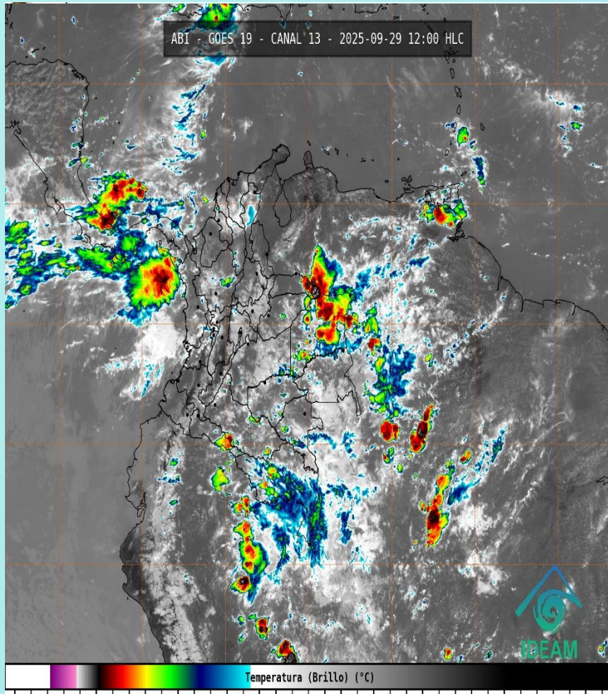
Imagen GOES 19 East Canal Infrarrojo, 29 de septiembre de 2025 - Hora 12:00 HLC. IDEAM – GOES 19
