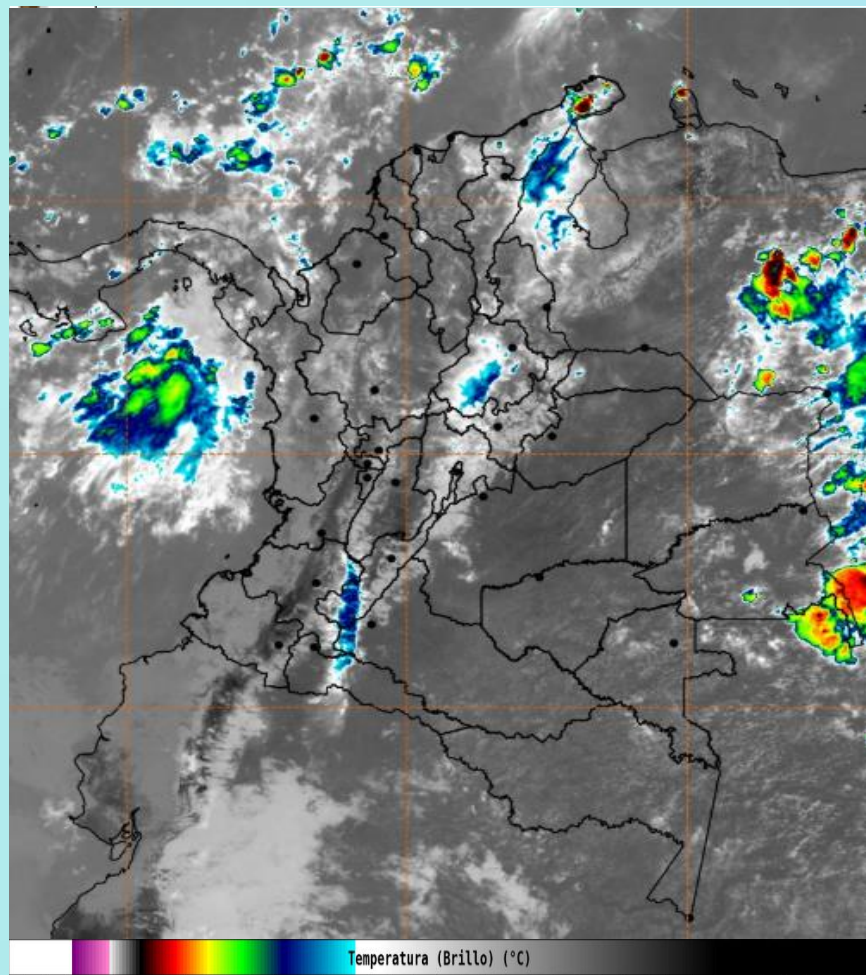
Imagen GOES 19 East Canal Infrarrojo, 27 de septiembre de 2025 - Hora 12:00 HLC. IDEAM – GOES 19
