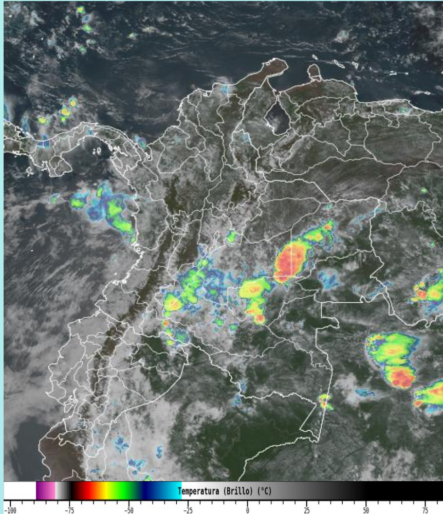
Imagen GOES 19 East Canal Infrarrojo, 23 de septiembre de 2025 - Hora 11:30 HLC. Fuente: https://rammb-slider.cira.colostate.edu/
