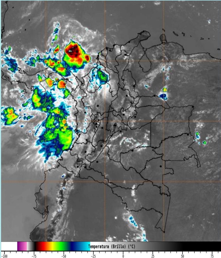
Imagen GOES 19 East Canal Infrarrojo, 21 de septiembre de 2025 - Hora 16:40 HLC. Fuente: IDEAM
