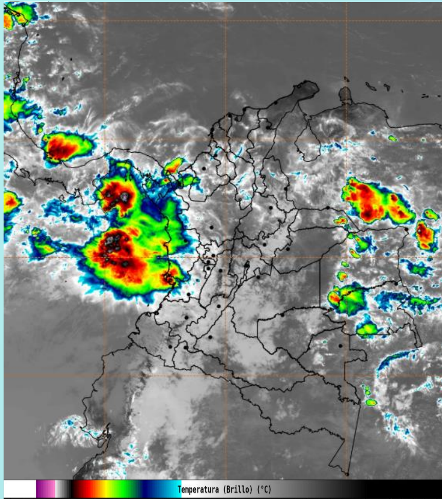
Imagen GOES 19 East Canal Infrarrojo, 11 de septiembre de 2025 - Hora 12:00 HLC. Fuente: IDEAM
