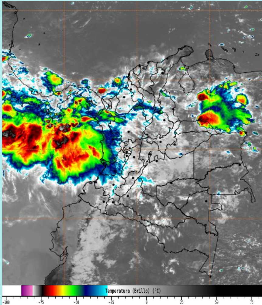
Imagen GOES 19 East Canal Infrarrojo, 4 de septiembre de 2025 - Hora 12:00 HLC. Fuente: IDEAM
