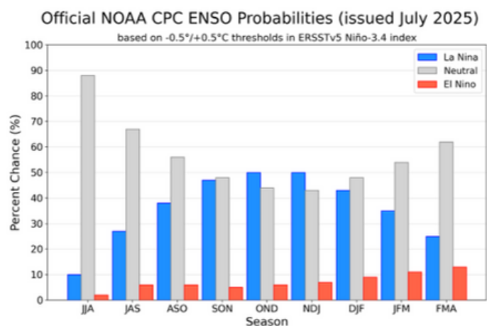
Figura 2: Pronóstico probabilístico del ENSO CPC/IRI. Fuente: CPC-IRI, publicado en julio 2025
