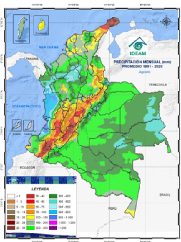
Figura 3: Climatología agosto
