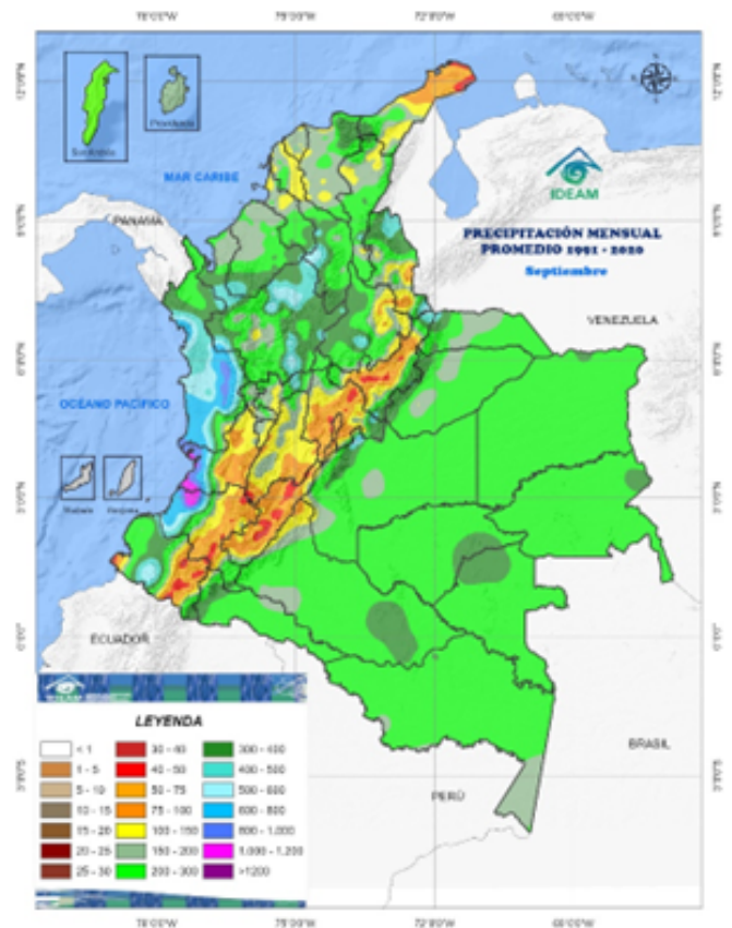
Figura 5: Climatología septiembre
