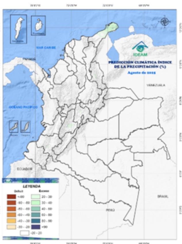
Figura 4: Predicción lluvias agosto
