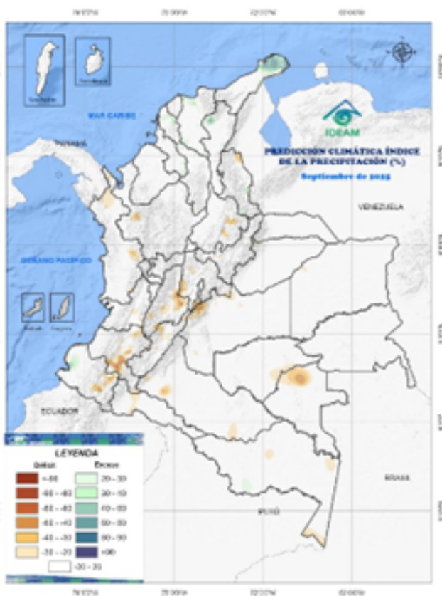
Figura 6: predicción de lluvias septiembre
