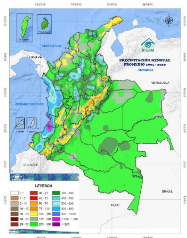
Figura 7: Climatología octubre
