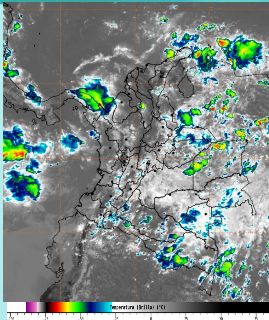
Imagen GOES 19 East Canal Infrarrojo, 8 de agosto de 2025 - Hora 12:00 HLC. Fuente: IDEAM
