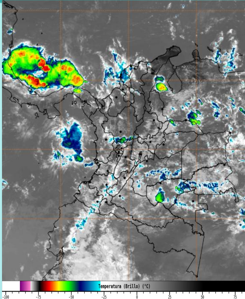
Imagen GOES 19 East Canal Infrarrojo, 6 de agosto de 2025 - Hora 12:00 HLC. Fuente: IDEAM
