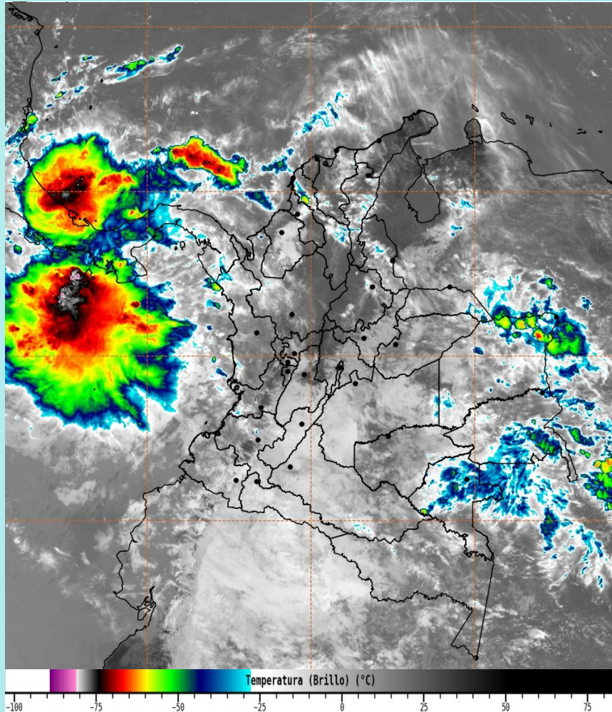
Imagen GOES 19 East Canal Infrarrojo, 3 de agosto de 2025 - Hora 11:40 HLC. Fuente: IDEAM
