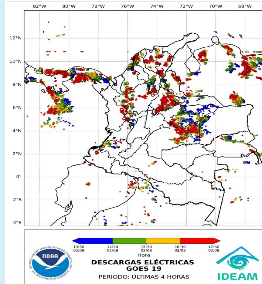
Descargas eléctricas (últimas horas) 2 de agosto de 2025 – Hora 17:30 HLC Fuente: NOAA - IDEAM
