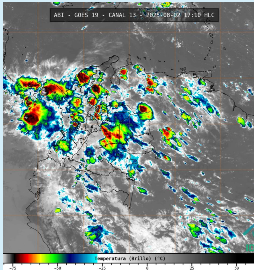
Imagen GOES 19 (East) Canal Infrarrojo 2 de agosto de 2025 – Hora 17:10 HLC Fuente: IDEAM – GOES 19
