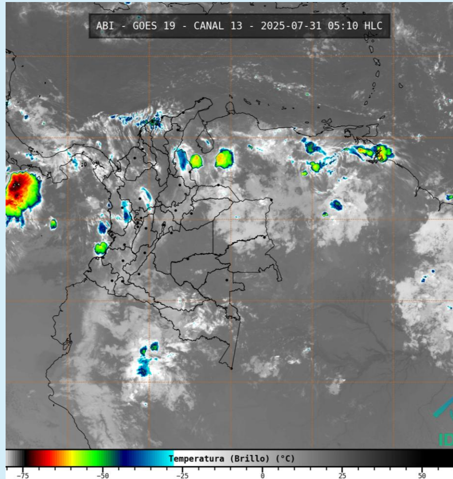
Imagen GOES 19 (East) Canal Infrarrojo 31 de julio de 2025 – Hora 05:10 HLC Fuente: IDEAM – GOES 19
