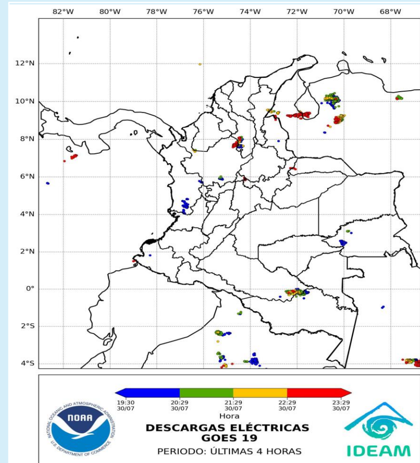
Descargas eléctricas (últimas horas) 30 de julio de 2025 – Hora 23:29 HLC Fuente: NOAA - IDEAM
