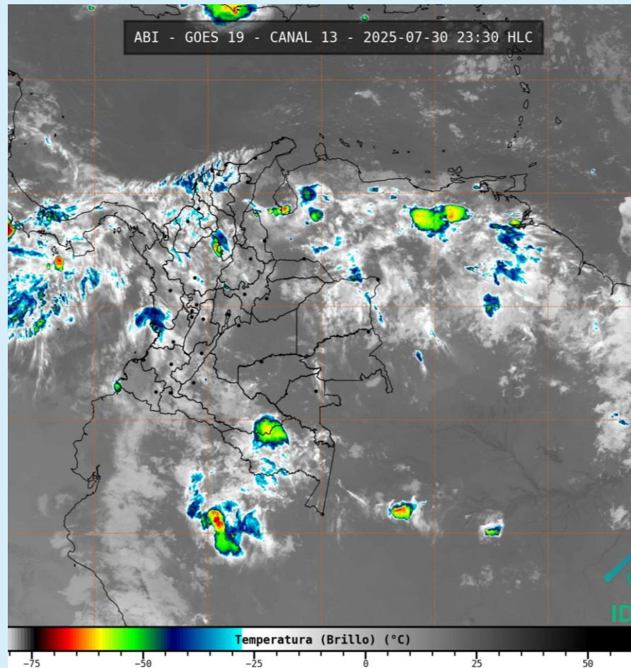
Imagen GOES 19 (East) Canal Infrarrojo 30 de julio de 2025 – Hora 23:30 HLC Fuente: IDEAM – GOES 19
