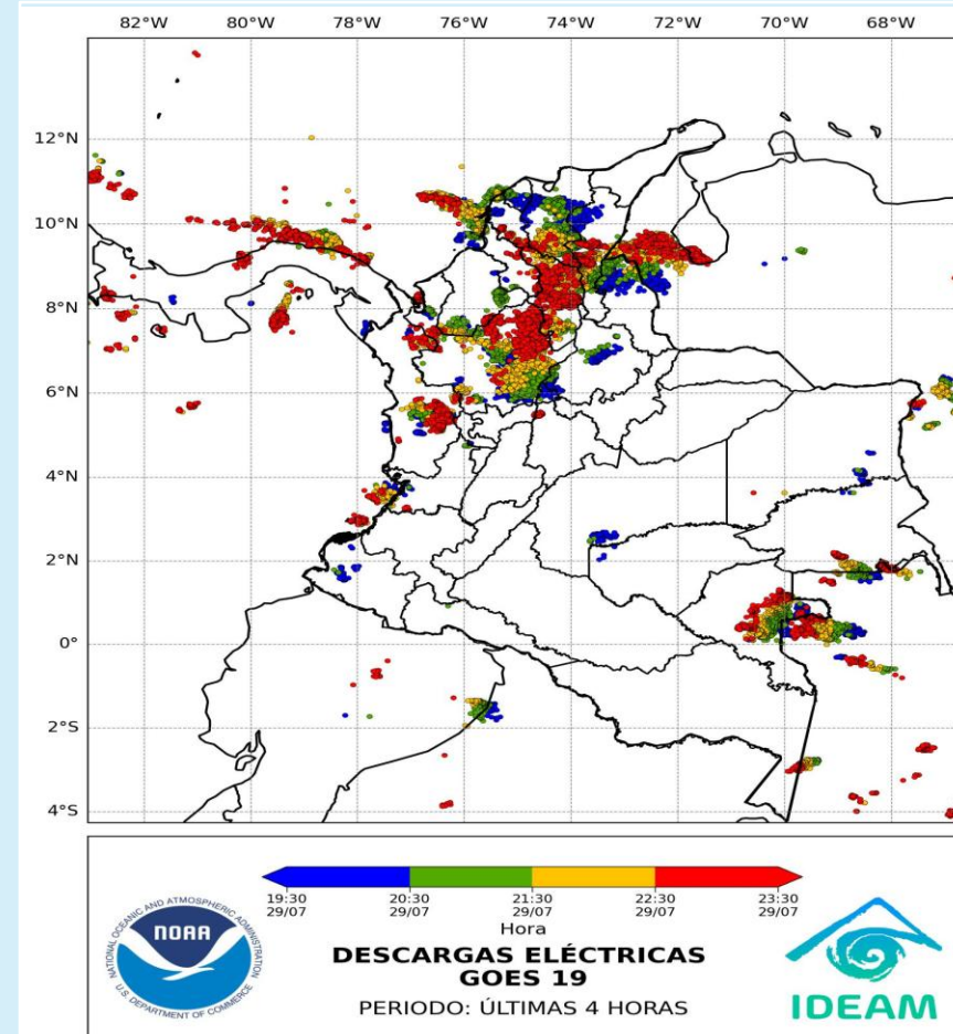
Descargas eléctricas (últimas horas) 29 de julio de 2025 – Hora 23:30 HLC Fuente: NOAA - IDEAM
