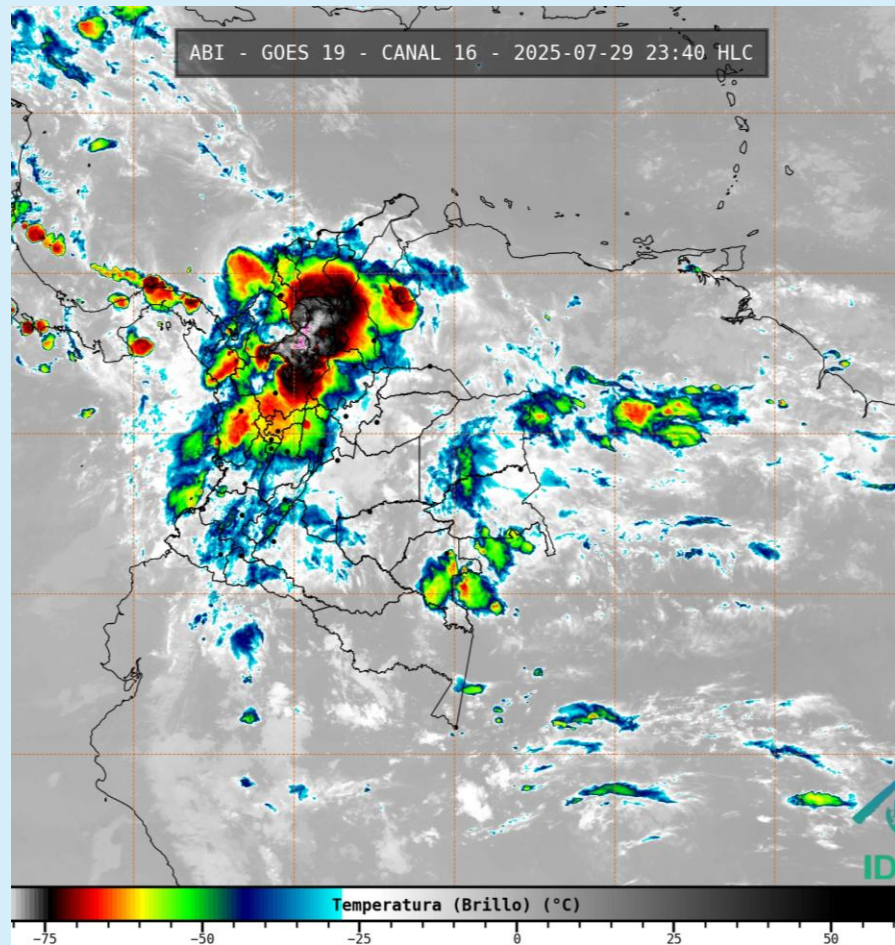
Imagen GOES 19 (East) Canal Infrarrojo 29 de julio de 2025 – Hora 23:40 HLC Fuente: IDEAM – GOES 19
