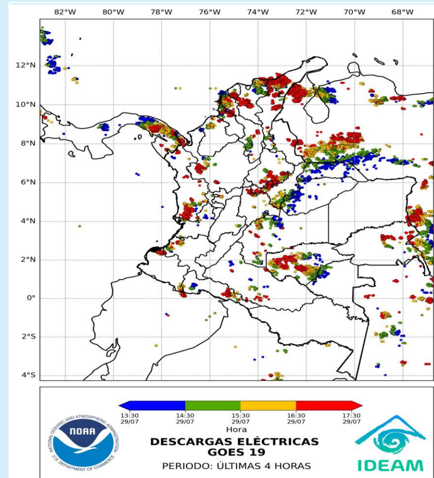
Descargas eléctricas (últimas horas) 29 de julio de 2025 – Hora 17:10 HLC Fuente: NOAA - IDEAM
