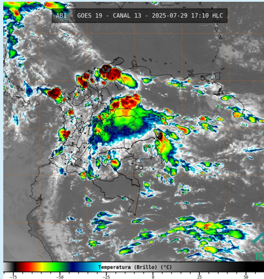
Imagen GOES 19 (East) Canal Infrarrojo 29 de julio de 2025 – Hora 17:10 HLC Fuente: IDEAM – GOES 19
