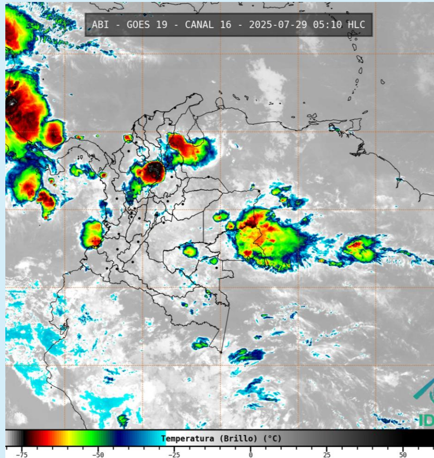
Imagen GOES 19 (East) Canal Infrarrojo 29 de julio de 2025 – Hora 05:10 HLC Fuente: IDEAM – GOES 19
