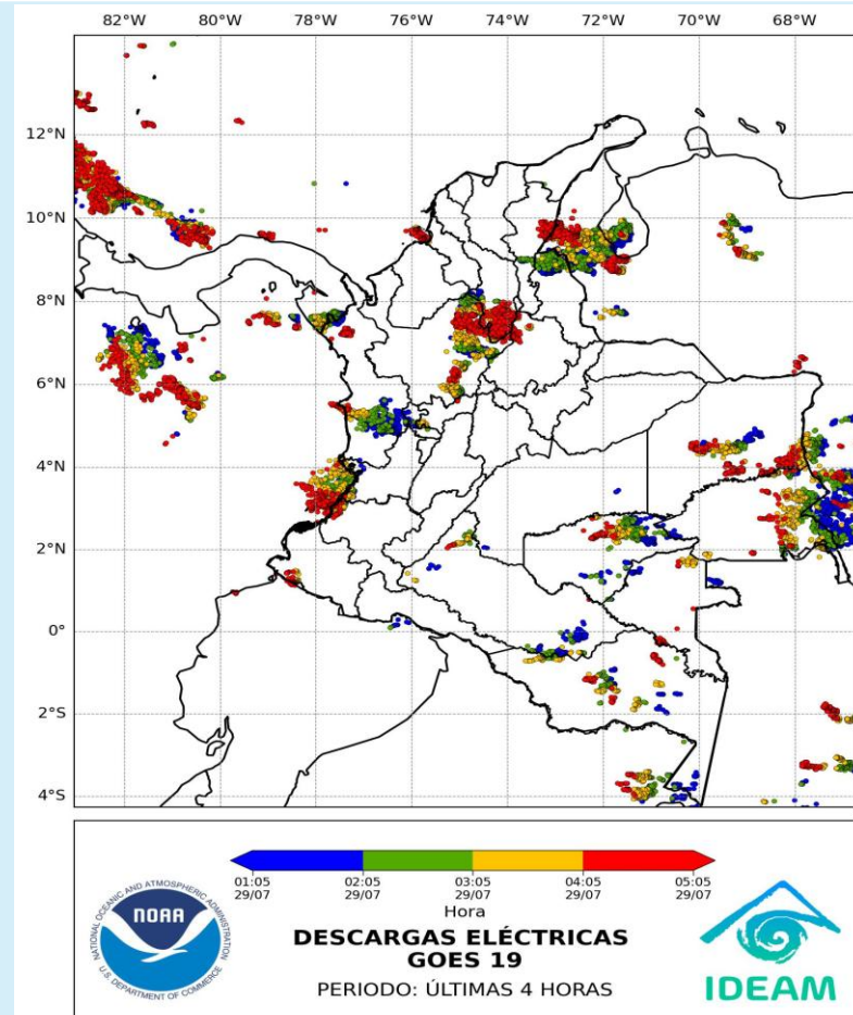
Descargas eléctricas (últimas horas) 29 de julio de 2025 – Hora 05:05 HLC Fuente: NOAA - IDEAM
