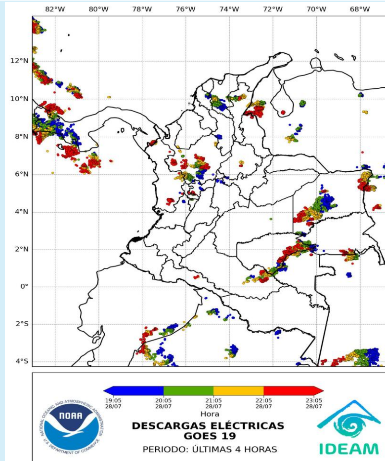
Descargas eléctricas (últimas horas) 28 de julio de 2025 – Hora 23:05 HLC Fuente: NOAA - IDEAM
