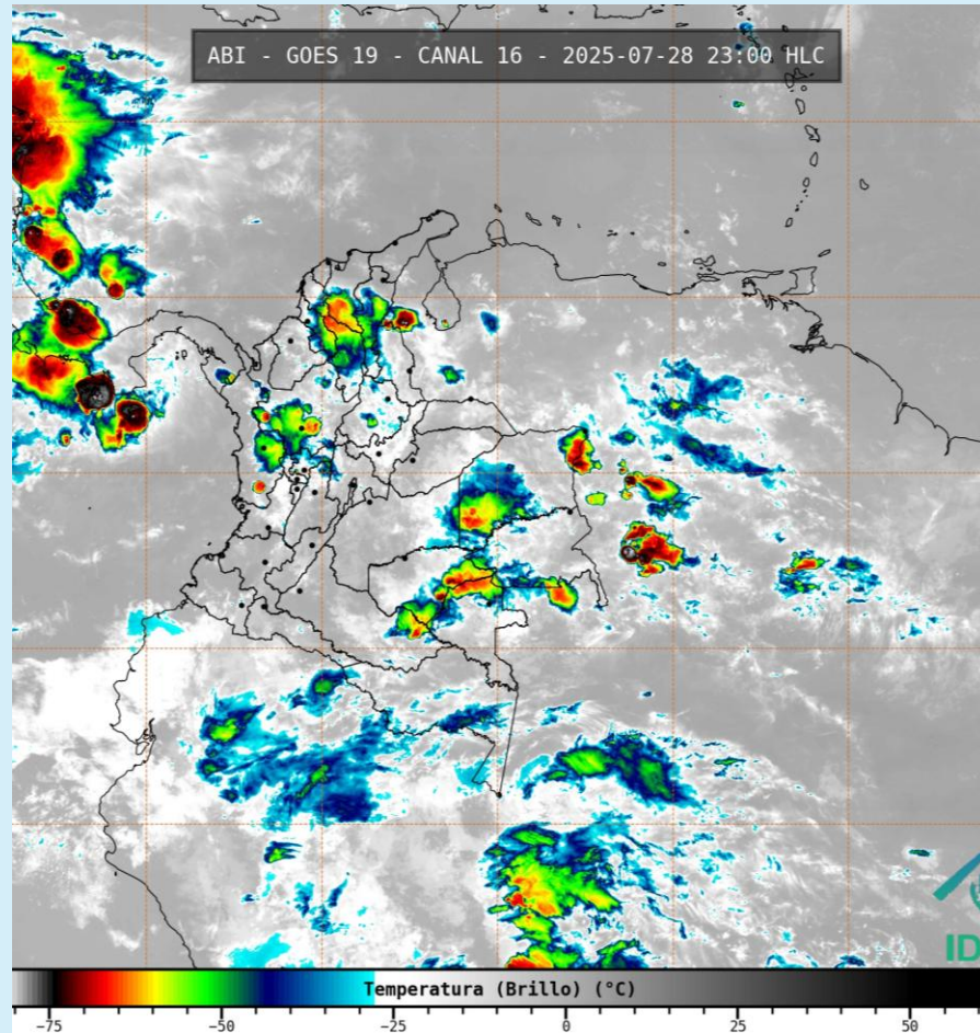
Imagen GOES 19 (East) Canal Infrarrojo 28 de julio de 2025 – Hora 23:00 HLC Fuente: IDEAM – GOES 19
