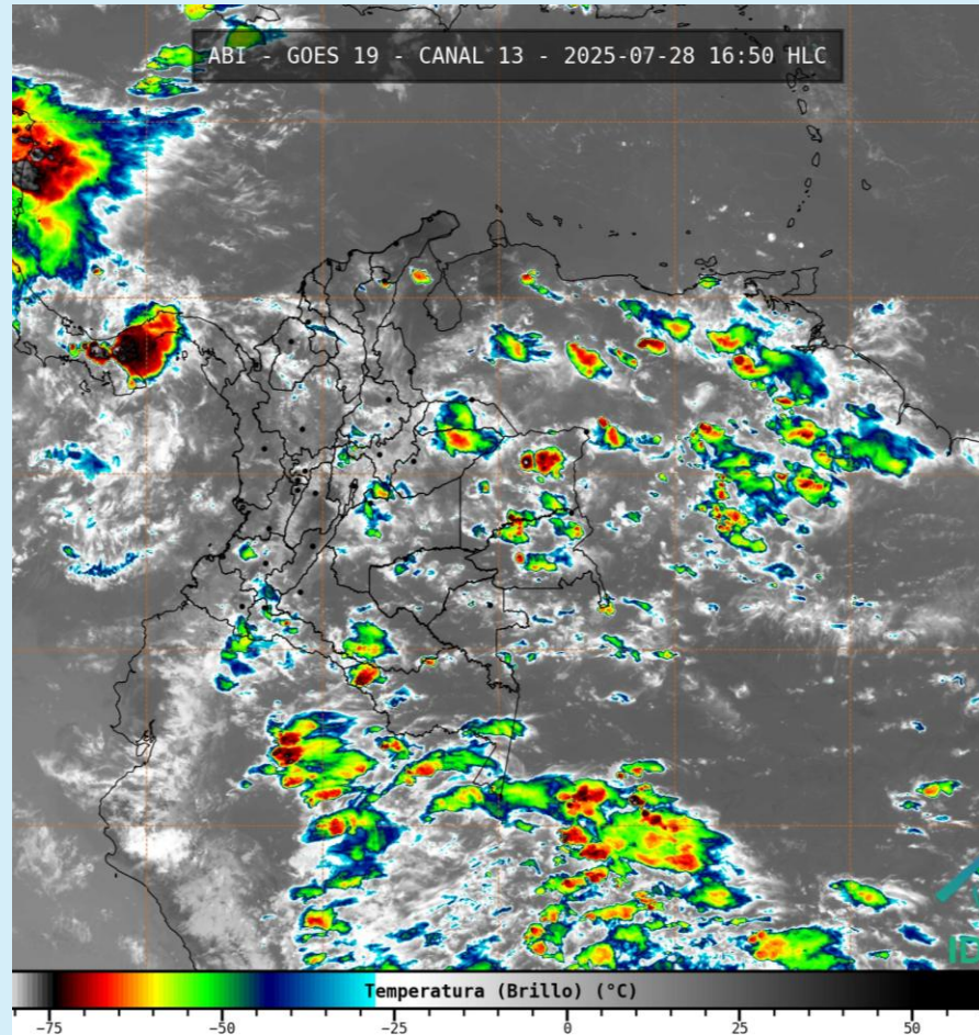
Imagen GOES 19 (East) Canal Infrarrojo 28 de julio de 2025 – Hora 16:50 HLC Fuente: IDEAM – GOES 19
