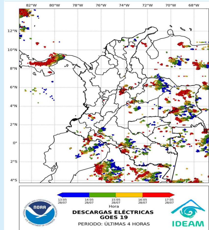
Descargas eléctricas (últimas horas) 28 de julio de 2025 – Hora 17:05 HLC Fuente: NOAA - IDEAM
