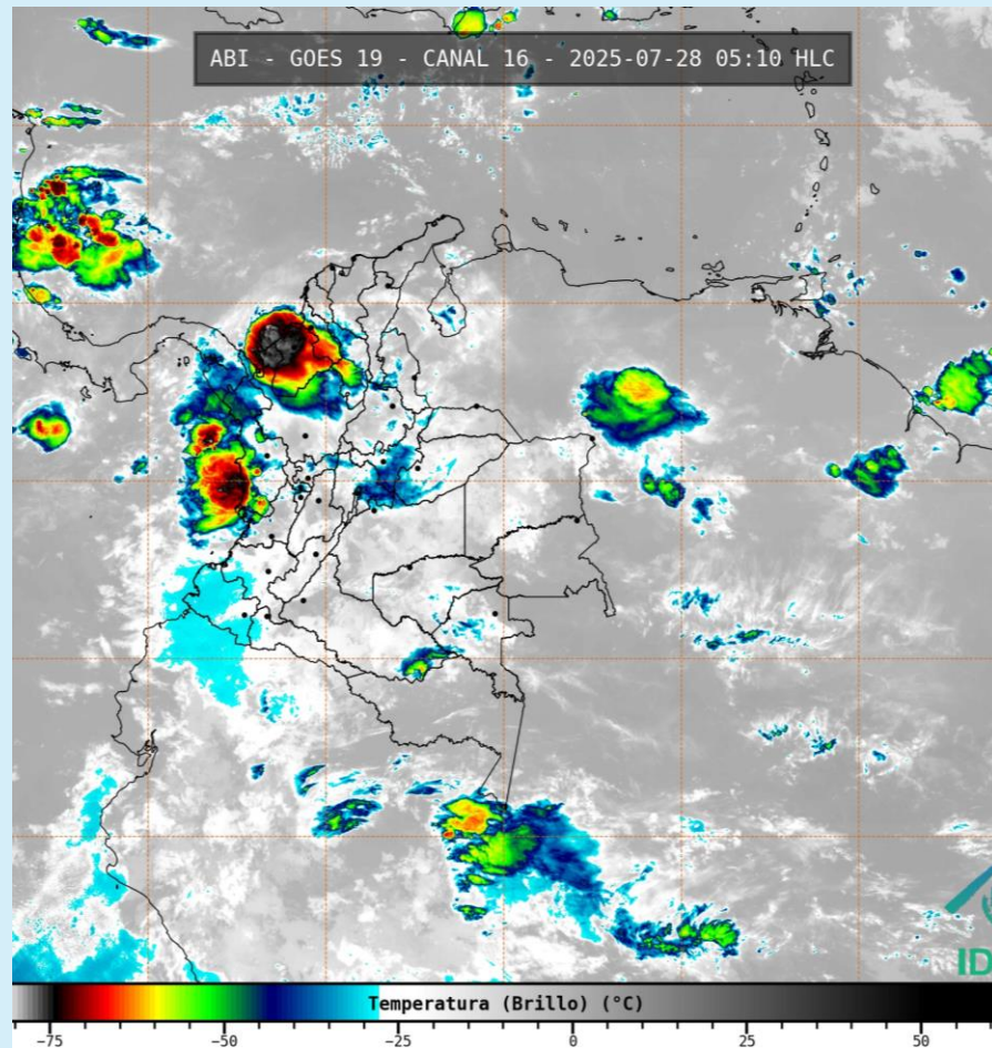
Imagen GOES 19 (East) Canal Infrarrojo 28 de julio de 2025 – Hora 05:10 HLC Fuente: IDEAM – GOES 19
