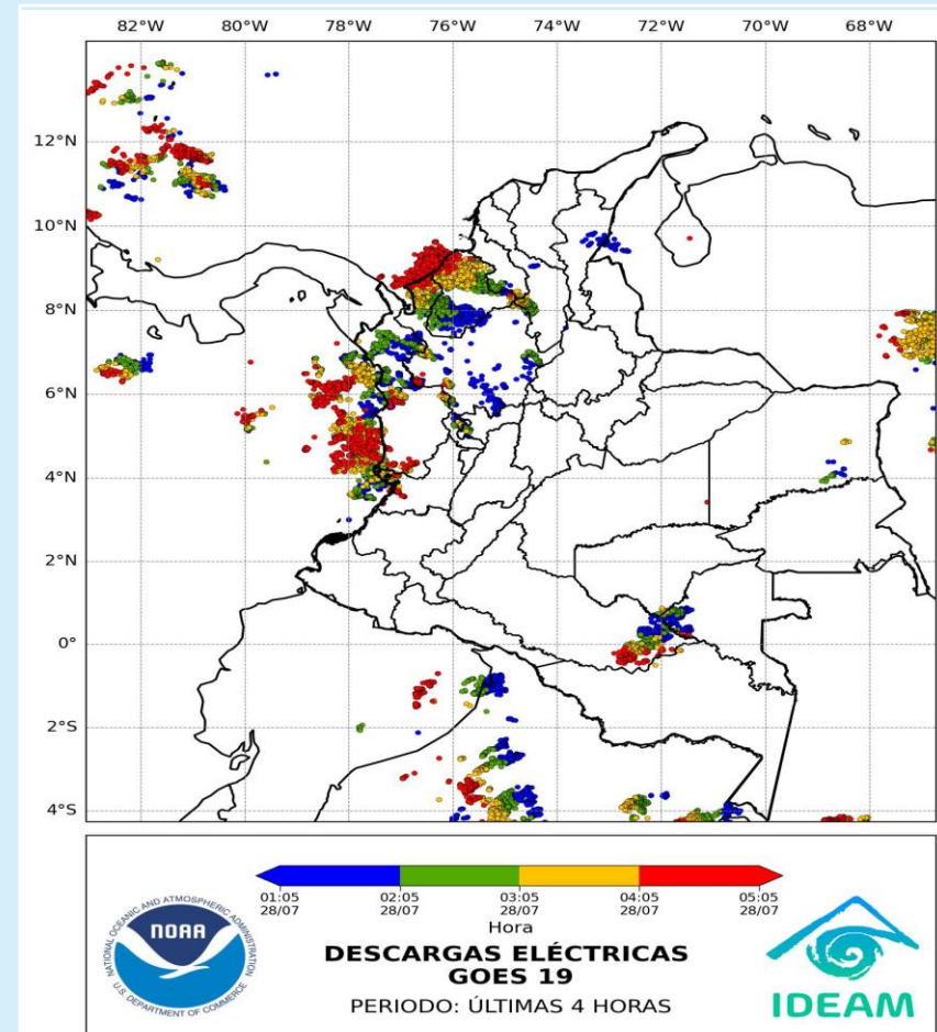
Descargas eléctricas (últimas horas) 28 de julio de 2025 – Hora 05:05 HLC Fuente: NOAA - IDEAM
