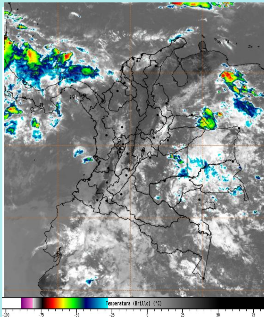
Imagen GOES 19 East Canal Infrarrojo, 27 de julio de 2025 - Hora 12:00 HLC. Fuente: rammb-slider.cira.colostate.edu
