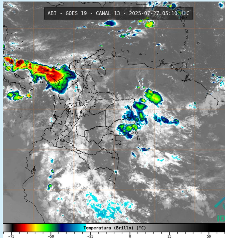
Imagen GOES 19 (East) Canal Infrarrojo 27 de julio de 2025 – Hora 05:10 HLC Fuente: IDEAM – GOES 19
