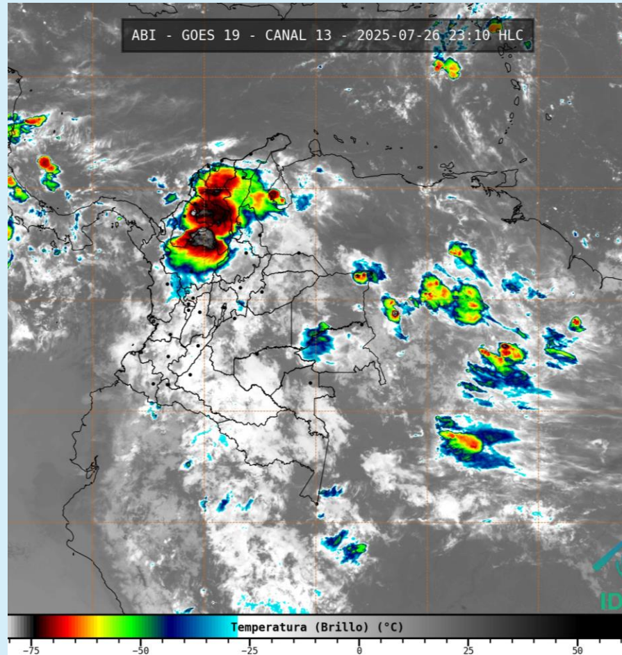
Imagen GOES 19 (East) Canal Infrarrojo 26 de julio de 2025 – Hora 23:10 HLC Fuente: IDEAM – GOES 19
