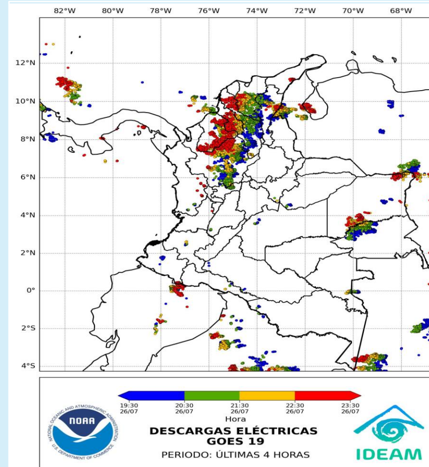
Descargas eléctricas (últimas horas) 26 de julio de 2025 – Hora 23:30 HLC Fuente: NOAA - IDEAM
