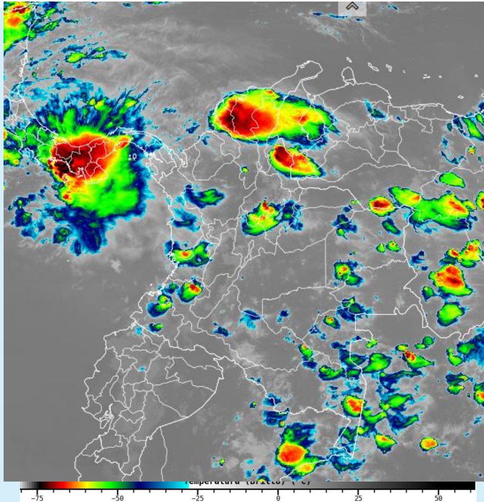
Imagen GOES 19 (East) Canal Infrarrojo 26 de julio de 2025 – Hora 06:00 HLC Fuente: IDEAM – GOES 19
