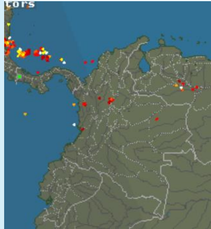
Descargas eléctricas (últimas horas) 26 de julio de 2025 – Hora 06:00 HLC Fuente: NOAA - IDEAM
