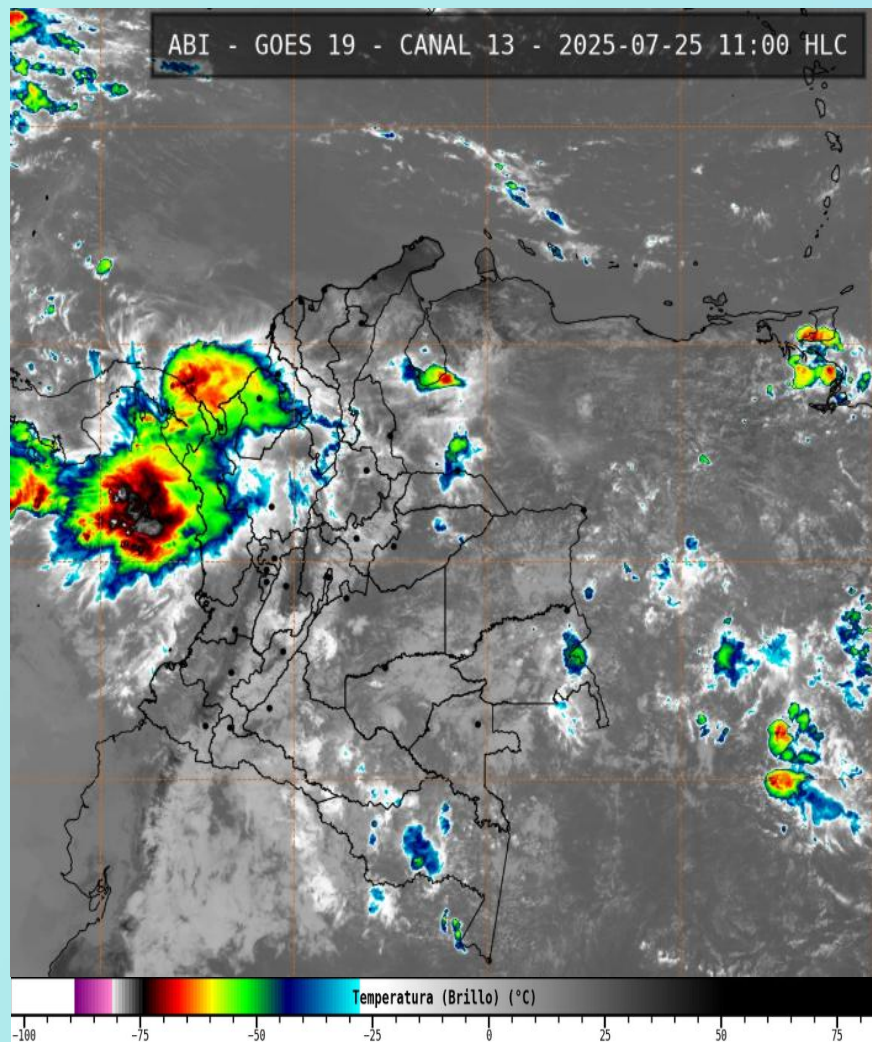
Imagen GOES 19 East Canal Infrarrojo, 25 de julio de 2025 - Hora 11:00 HLC. Fuente: rammb-slider.cira.colostate.edu
