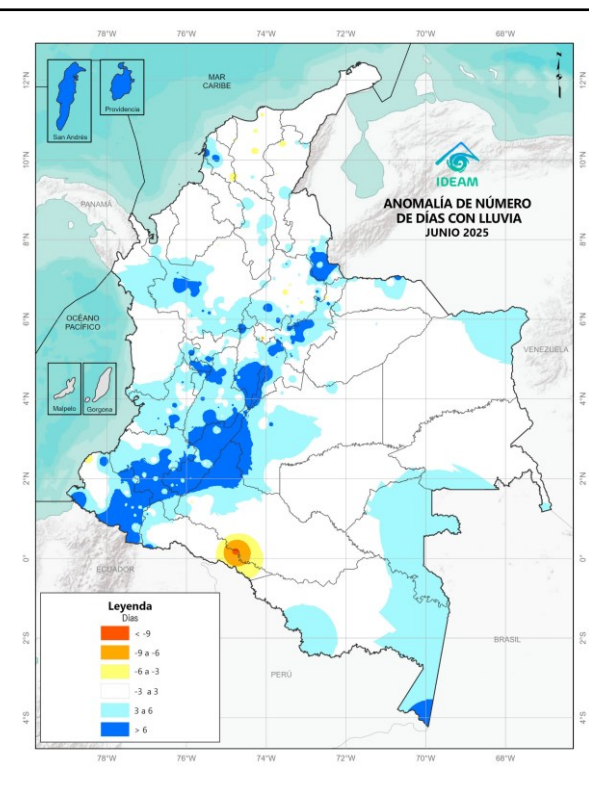
Anomalia de número de días con lluvia
