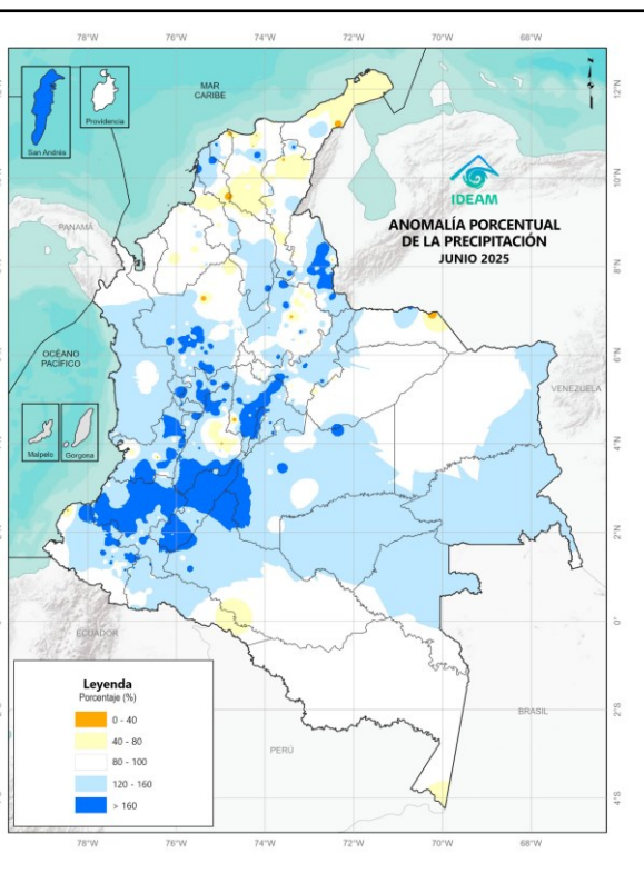
Anomalia porcentual de la precipitación (%)
