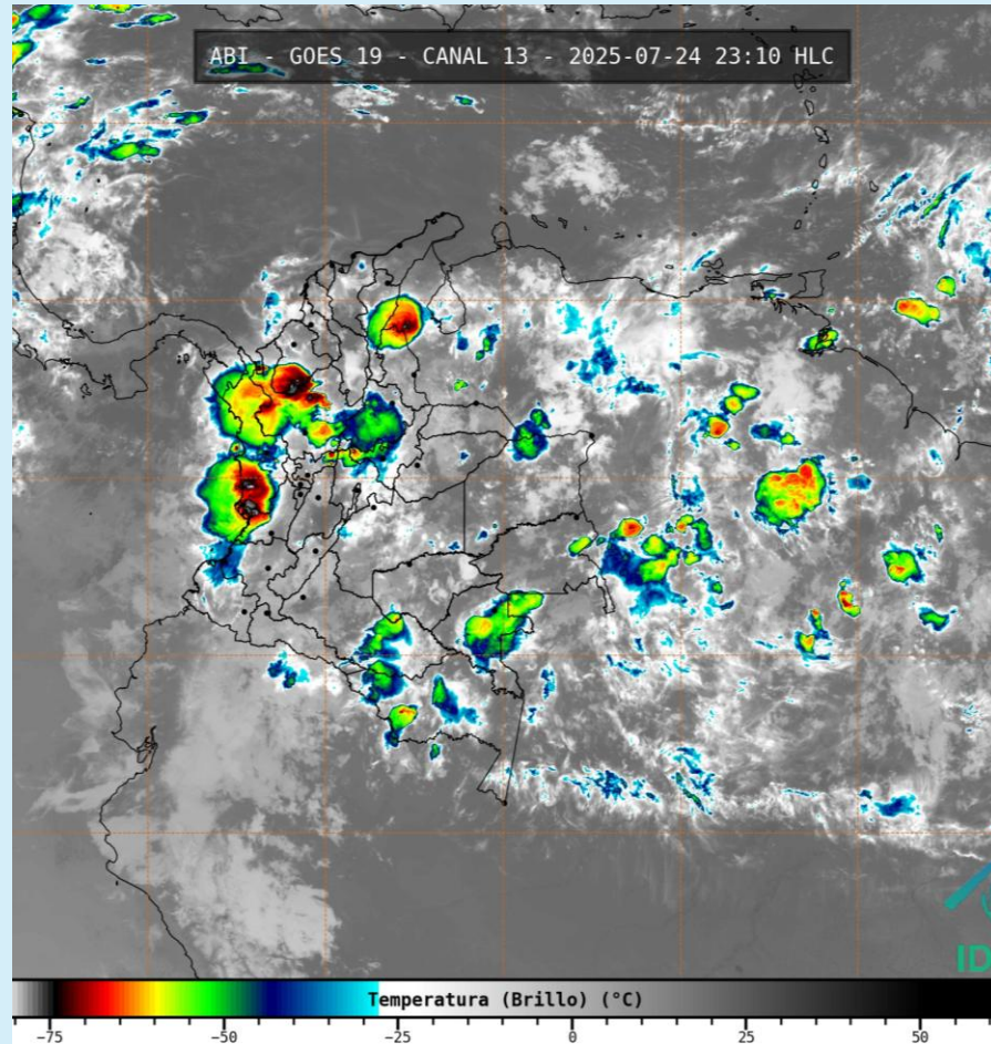
Imagen GOES 19 (East) Canal Infrarrojo 24 de julio de 2025 – Hora 23:10 HLC Fuente: IDEAM – GOES 19
