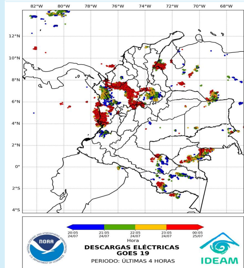
Descargas eléctricas (últimas horas) 25 de julio de 2025 – Hora 00:05 HLC Fuente: NOAA - IDEAM
