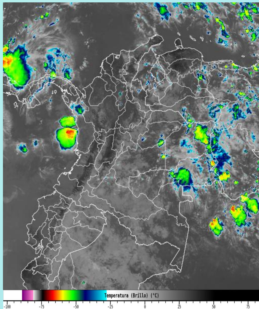
Imagen GOES 19 East Canal Infrarrojo, 24 de julio de 2025 - Hora 11:30 HLC. Fuente: rammb-slider.cira.colostate.edu
