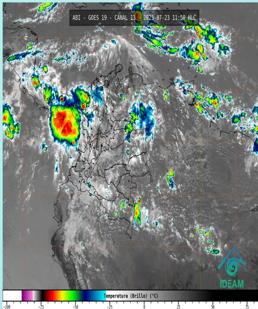
Imagen GOES 19 East Canal Infrarrojo, 23 de julio de 2025 - Hora 11:50 HLC. Fuente: IDEAM
