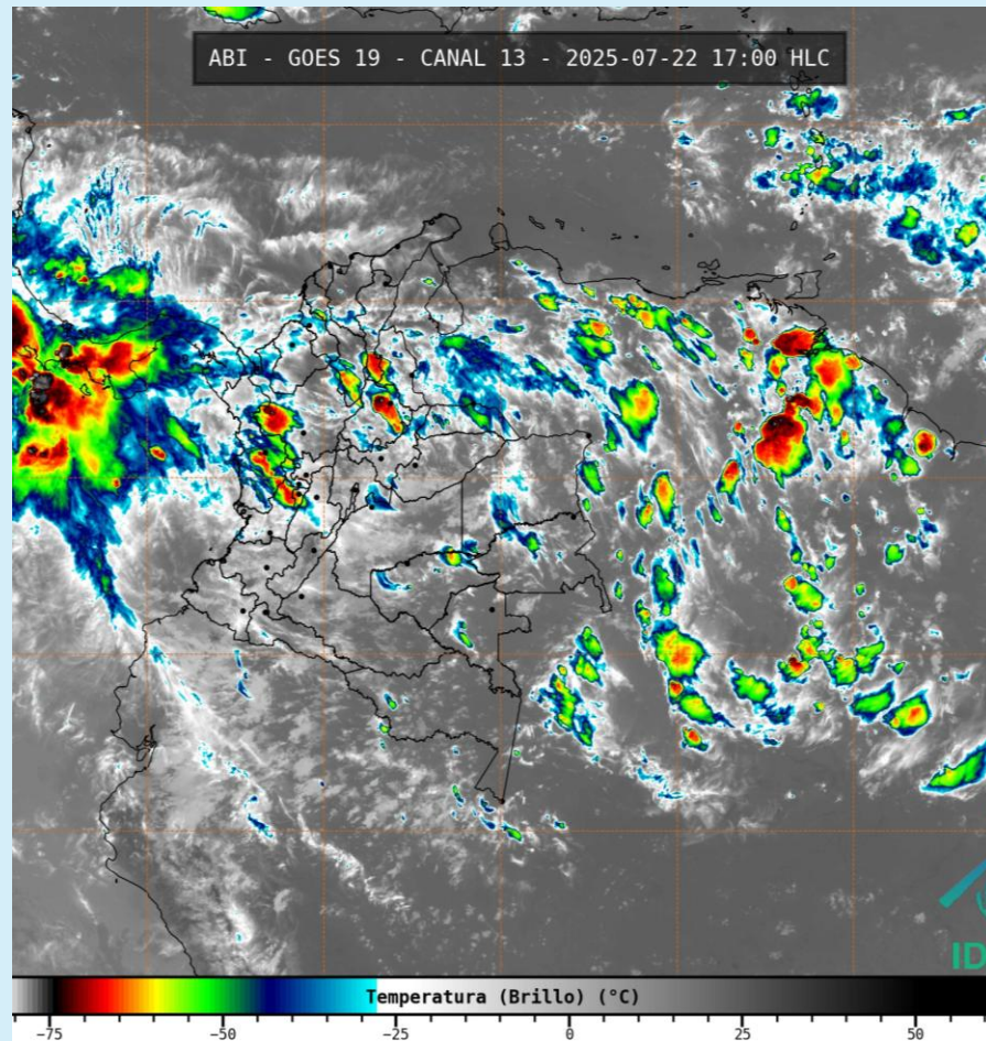
Imagen GOES 19 (East) Canal Infrarrojo 22 de julio de 2025 – Hora 17:00 HLC Fuente: IDEAM – GOES 19
