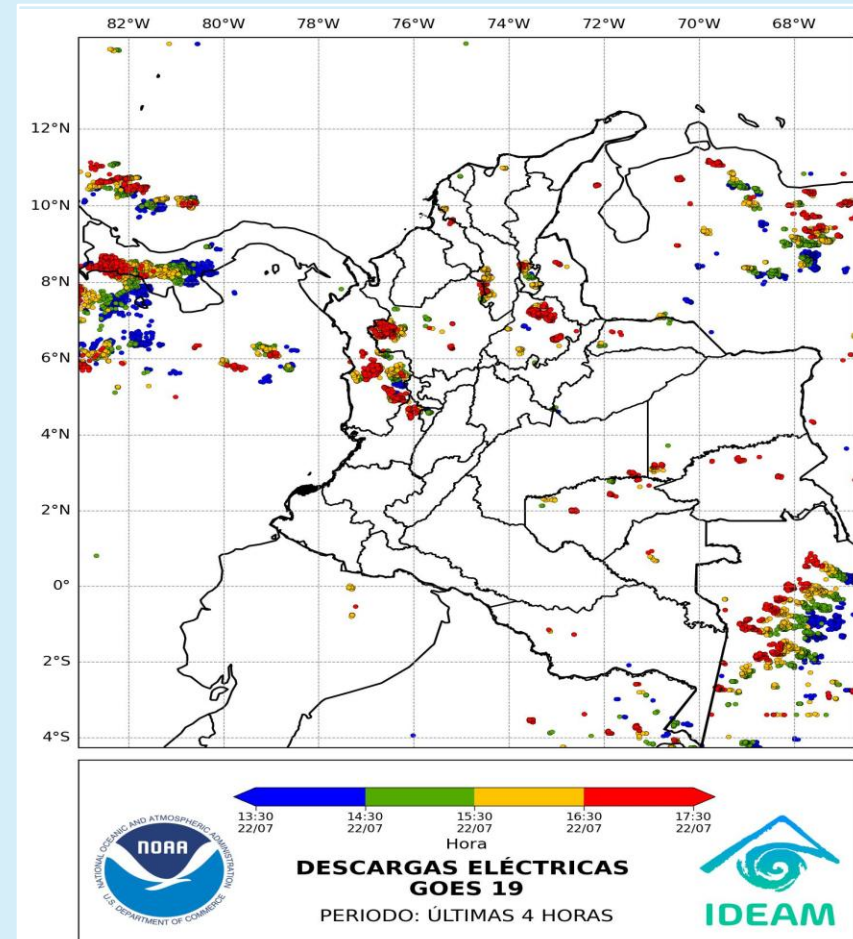
Descargas eléctricas (últimas horas) 22 de julio de 2025 – Hora 17:00 HLC Fuente: NOAA - IDEAM
