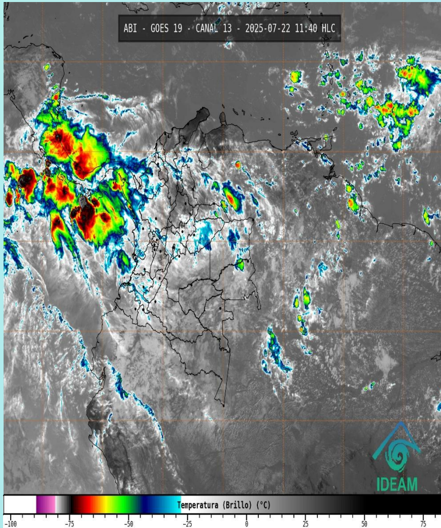
Imagen GOES East Canal Infrarrojo, 22 de julio de 2025 - Hora 11:40 HLC. Fuente: IDEAM
