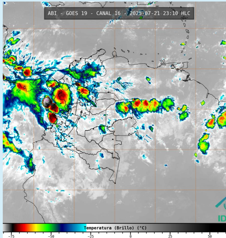
Imagen GOES 19 (East) Canal Infrarrojo 21 de julio de 2025 - Hora 23:10 HLC Fuente: IDEAM – GOES 19
