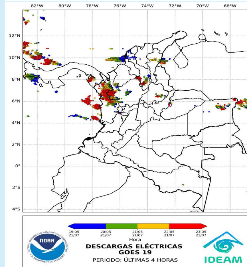
Descargas eléctricas (últimas horas) 21 de julio de 2025 – Hora 23:05 HLC Fuente: NOAA - IDEAM
