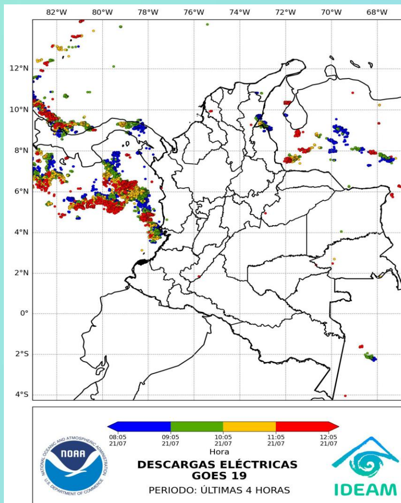
Descargas eléctricas en las últimas cuatro horas. Hora 12:05 HLC Fuente: IDEAM
