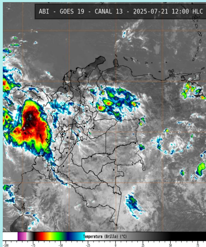
Imagen GOES East Canal Infrarrojo, 21 de julio de 2025 - Hora 12:00 HLC. Fuente: IDEAM
