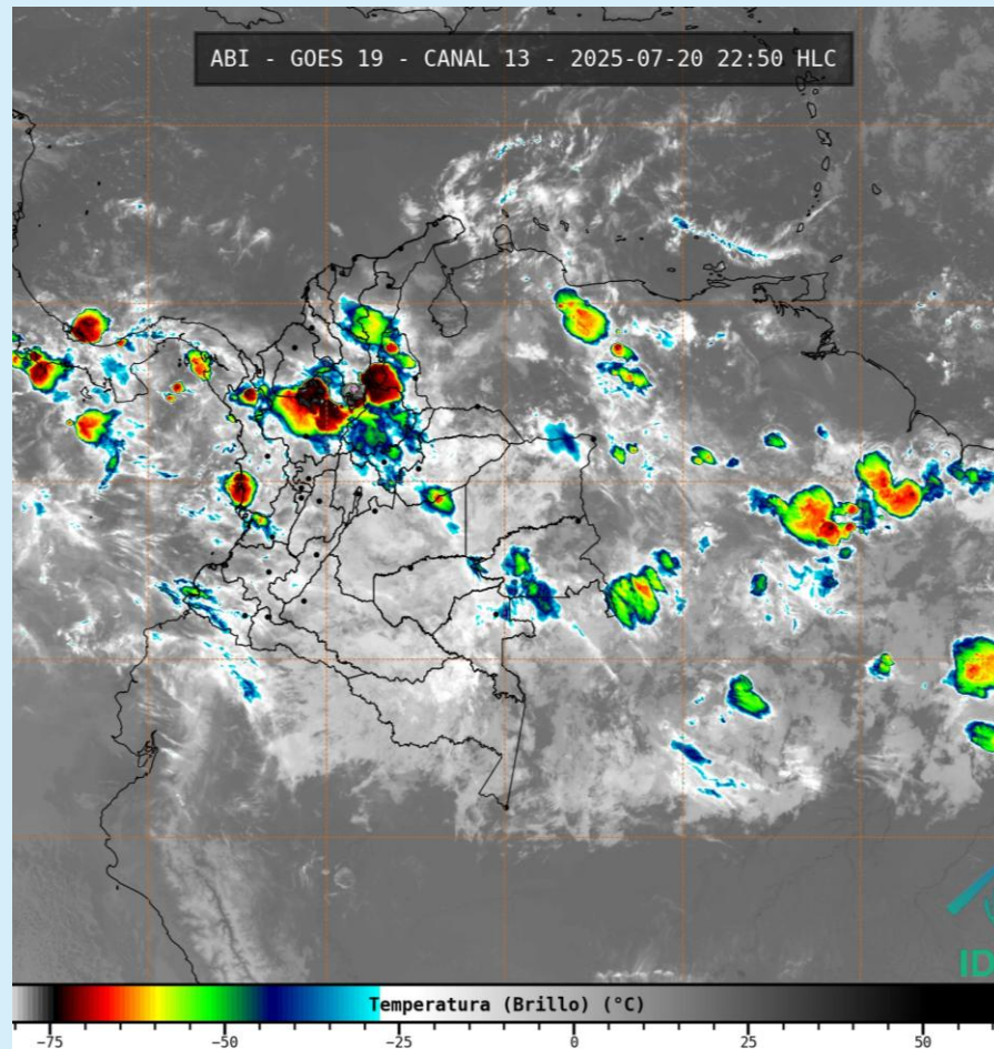
Imagen GOES 19 (East) Canal Infrarrojo 20 de julio de 2025 - Hora 22:50 HLC Fuente: IDEAM – GOES 19
