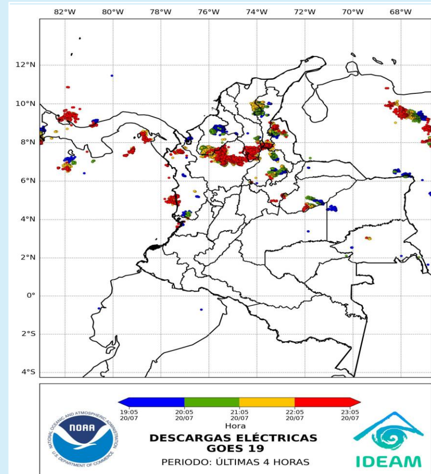
Descargas eléctricas (últimas horas) 20 de julio de 2025 – Hora 23:05 HLC Fuente: NOAA - IDEAM
