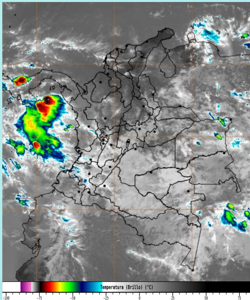
Imagen GOES East Canal Infrarrojo, 20 de julio de 2025 - Hora 11:30 HLC. Fuente: IDEAM
