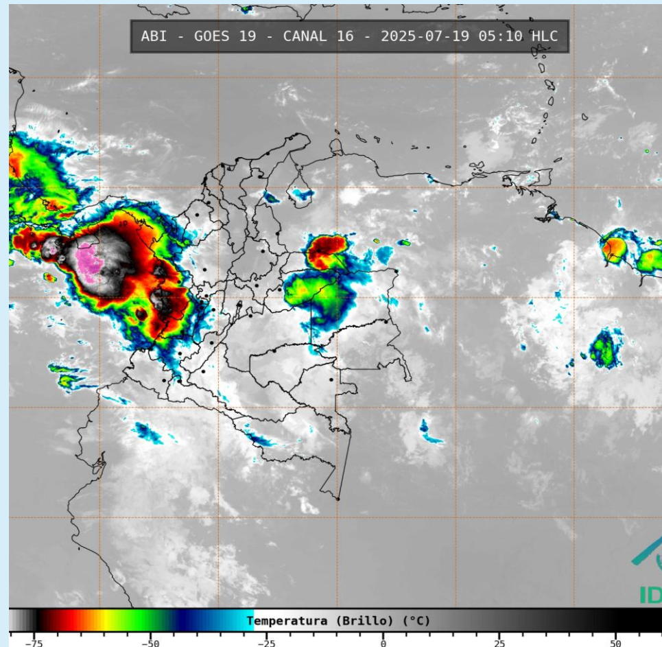
Imagen GOES 19 (East) Canal Infrarrojo 19 de julio de 2025 - Hora 05:10 HLC Fuente: IDEAM – GOES 19
