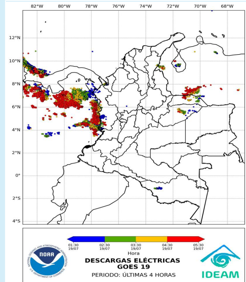
Descargas eléctricas (últimas horas) 19 de julio de 2025 – Hora 05:05 HLC Fuente: NOAA - IDEAM
