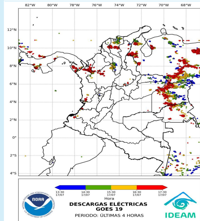
Descargas eléctricas (últimas horas) 17 de julio de 2025 – Hora 17:10 HLC Fuente: NOAA - IDEAM
