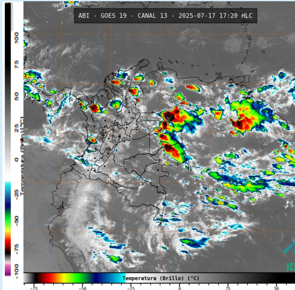
Imagen GOES 19 (East) Canal Infrarrojo 17 de julio de 2025 - Hora 17:20 HLC Fuente: IDEAM – GOES 19
