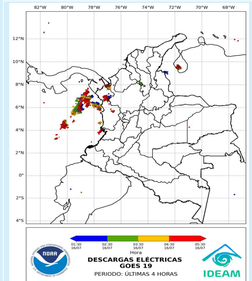
Descargas eléctricas (últimas horas) 16 de julio de 2025 – Hora 05:30 HLC Fuente: NOAA - IDEAM
