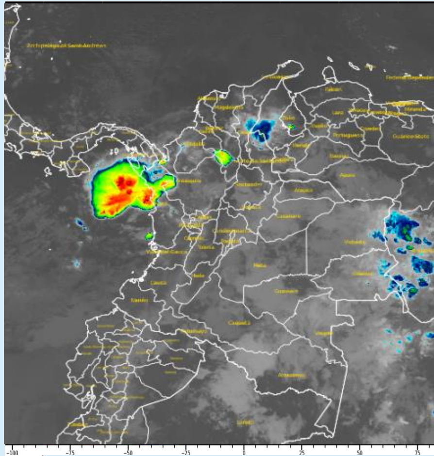
Imagen GOES 19 (East) Canal Infrarrojo 16 de julio de 2025 - Hora 05:10 HLC Fuente: RAMMB – GOES 19
