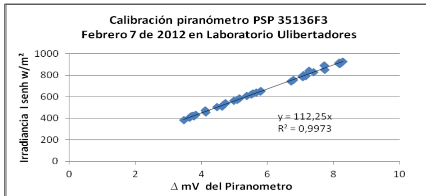
Figura 10. Gráfica de correlación de los valores de I senh contra \Delta mV . (Fuente: Fundación Universitaria Los Libertadores)
