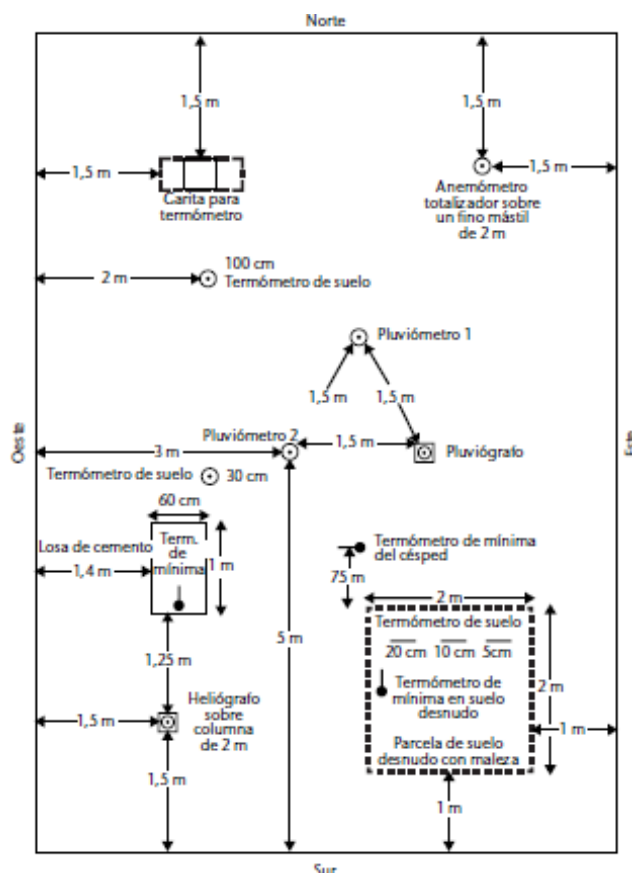
Figura 2. Disposición de una estación de observación en el hemisferio norte que muestra las distancias mínimas entre las instalaciones. Fuente: Tomado de OMM, 2010
