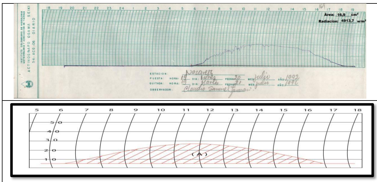
Figura 12. Gráfica de actinógrafo. Arriba gráfica del actinógrafo de la estación Nazareth en La Guajira para el 21 de julio de 1992. Abajo, área bajo la curva (Fuente: IDEAM)
