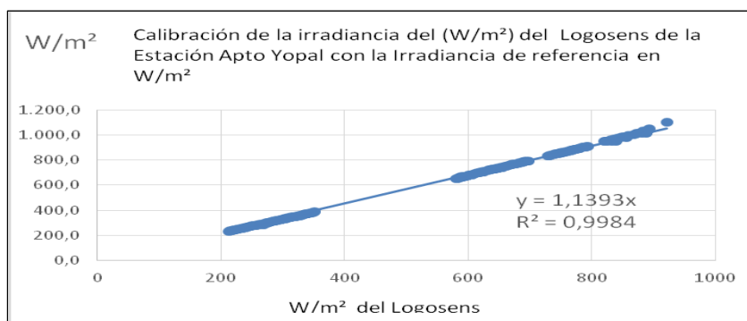
Figura 11. Gráfica de correlación entre la irradiancia del sensor de referencia y la del logosens de la estación del aeropuerto de Yopal en el año 2014. (Fuente: Fundación Universitaria Los Libertadores)
