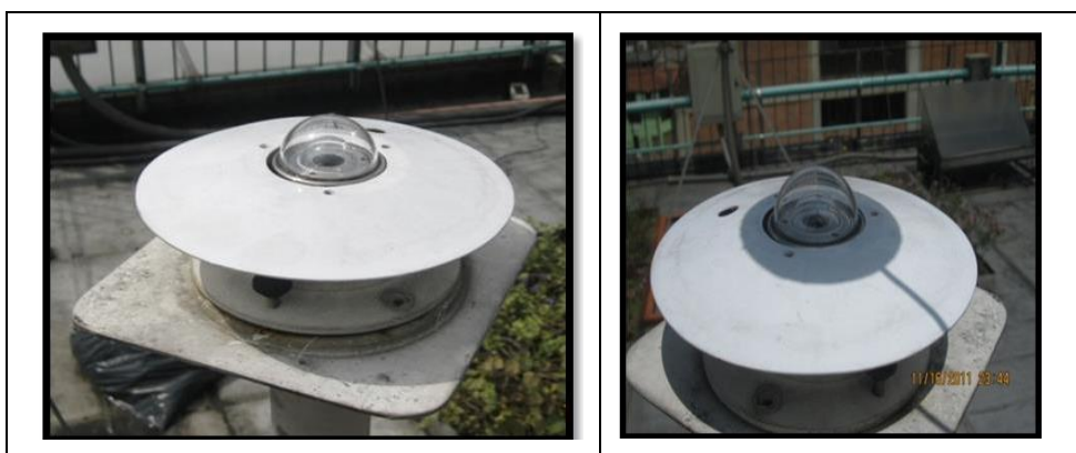
Figura 8. a) Piranómetro destapado (mide radiación global) y b) tapado (mide radiación difusa). (Fuente: Fundación Universitaria Los Libertadores)
