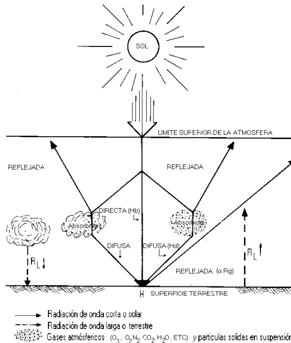
Figura 1. Atenuación de la radiación solar por la atmósfera terrestre.
