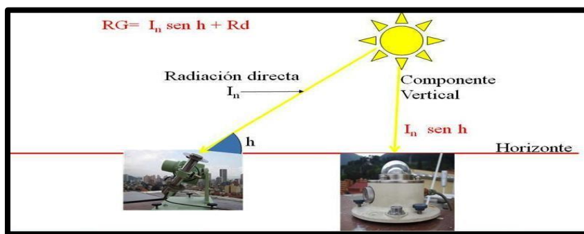
Figura 9. Geometría de los rayos solares. (Fuente: Fundación Universitaria Los Libertadores)
