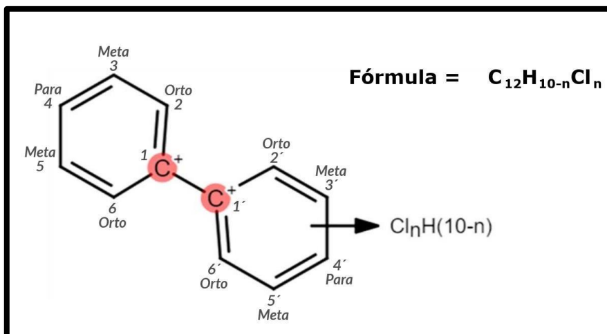
Figura 1. Posiciones que pueden adoptar los átomos de cloro sobre la molécula de PCB
