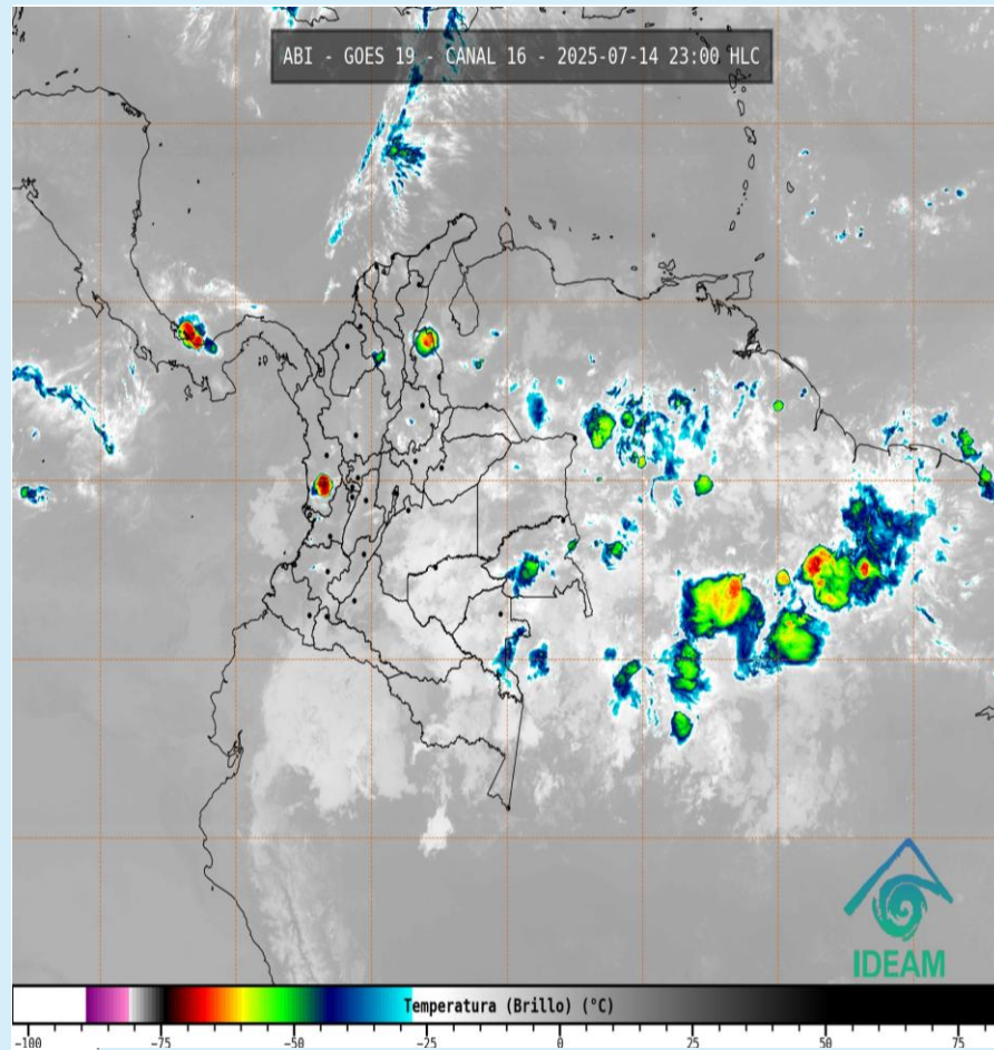
Imagen GOES 19 (East) Canal Infrarrojo 14 de julio de 2025 - Hora 23:00 HLC Fuente: RAMMB – GOES 19
