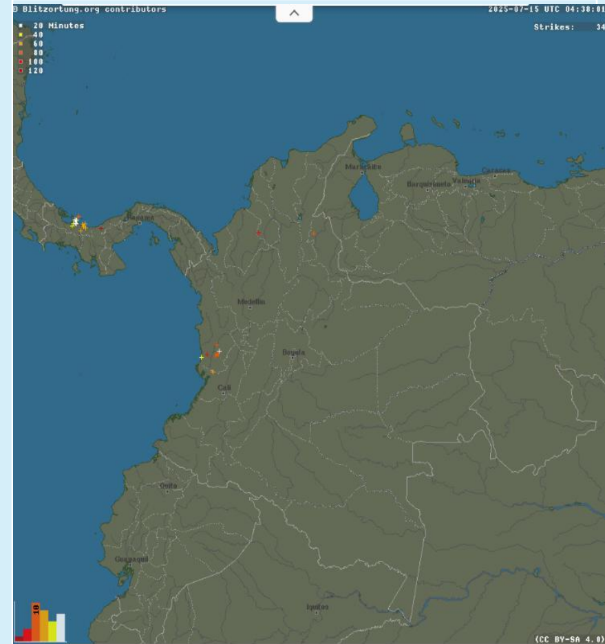
Descargas eléctricas (últimas horas) 14 de julio de 2025 – Hora 23:30 HLC Fuente: https://www.blitzortung.org/es/live_lightning_maps.php#google_vignette
