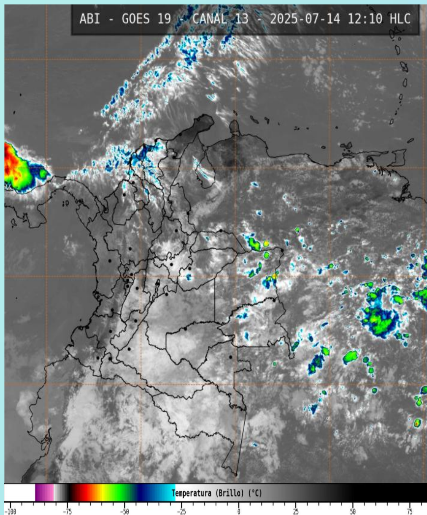
Imagen GOES East Canal Infrarrojo, 14 de julio de 2025 - Hora 12:10 HLC. Fuente: IDEAM
