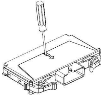
Figura 8. Retirar la cubierta del bloque terminal.
