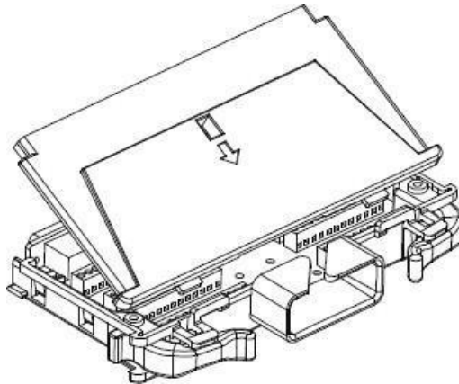
Figura 9. Retirar la tapa de plástico del bloque terminal.
