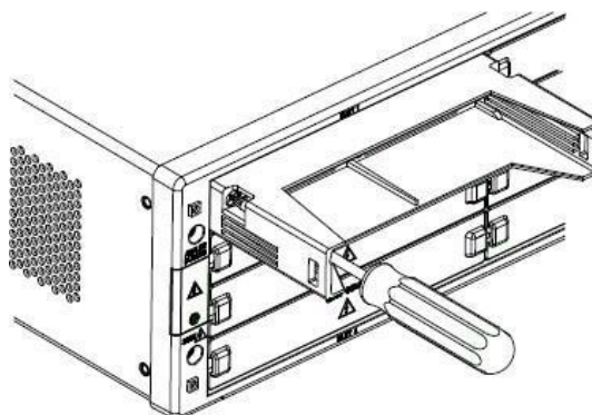
Figura 7. Instalación del módulo a la ranura.
