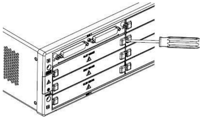
Figura 2. Procedimiento para retirar las cubiertas de las ranuras.
