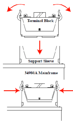
Figura 18. Anclaje del bloque terminal.
