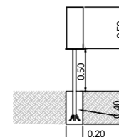
VISTA FRONTAL PLUVIOMETRO
