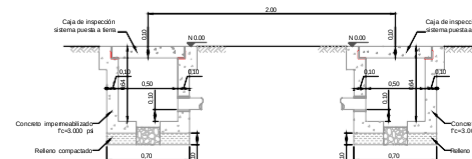
DETALLE CAJAS DE INSPECCIÓN POLO A TIERRA
