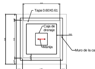
PLANTA CAJA DE INSPECCIÓN SISTEMA PUESTA A TIERRA
