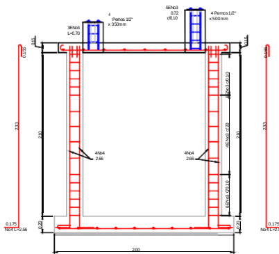
REFUERZO ESTRUCTURAL COLUMNAS
