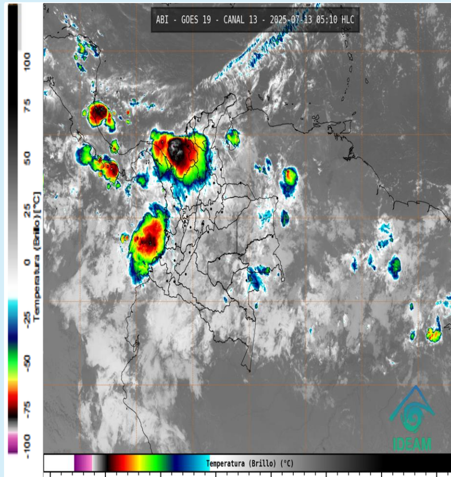
Imagen GOES 19 (East) Canal Infrarrojo 13 de julio de 2025 - Hora 05:10 HLC Fuente: RAMMB – GOES 19
