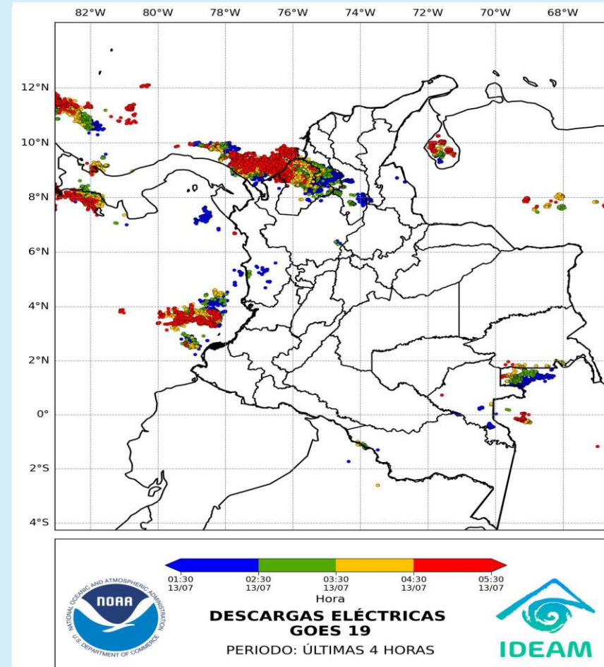
Descargas eléctricas (últimas horas) 13 de julio de 2025 – Hora 05:35 HLC Fuente: NOAA - IDEAM
