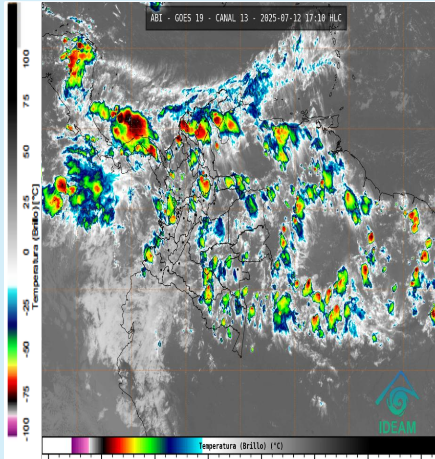
Imagen GOES 19 (East) Canal Infrarrojo 12 de julio de 2025 - Hora 17:10 HLC Fuente: RAMMB – GOES 19
