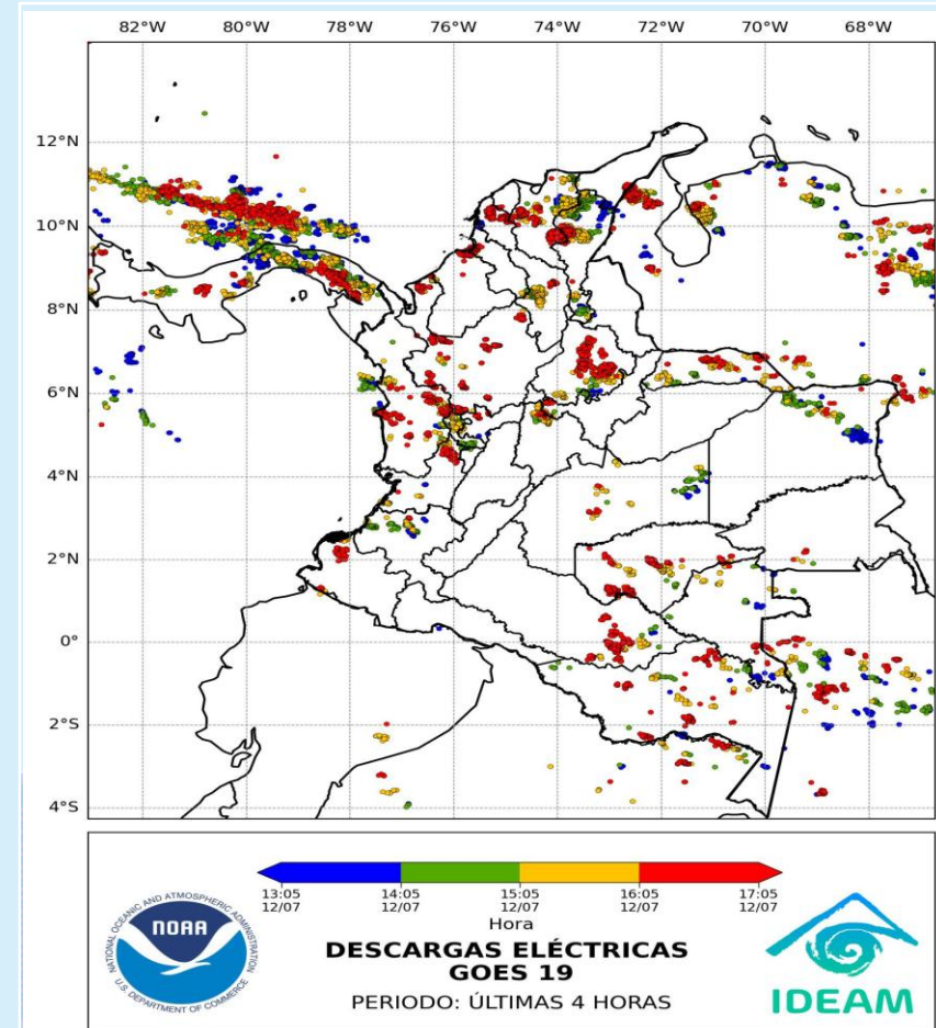
Descargas eléctricas (últimas horas) 12 de julio de 2025 – Hora 17:10 HLC Fuente: NOAA - IDEAM
