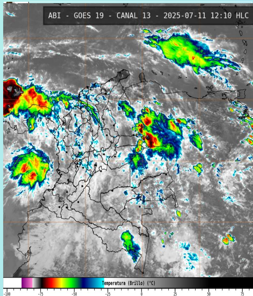
Imagen GOES East Canal Infrarrojo, 11 de julio de 2025 - Hora 12:10 HLC. Fuente: IDEAM
