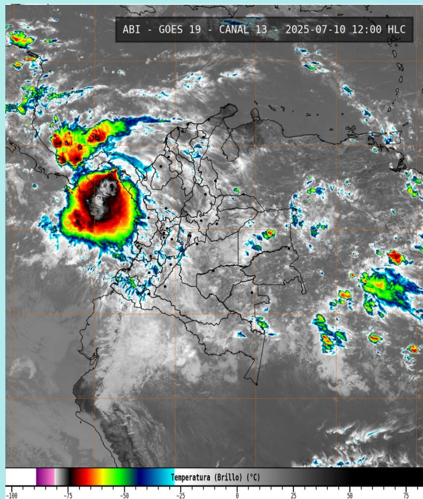
Imagen GOES East Canal Infrarrojo, 10 de julio de 2025 - Hora 12:00 HLC. Fuente: IDEAM
