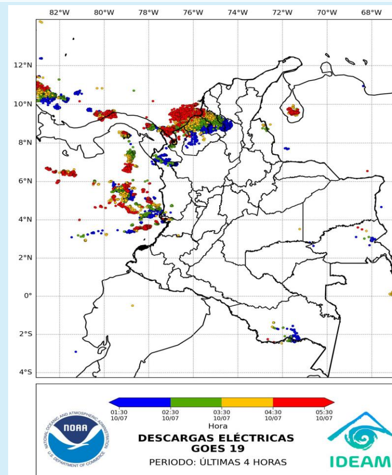
Descargas eléctricas 10 de julio de 2025 – Hora 05:30 HLC Fuente: IDEAM
