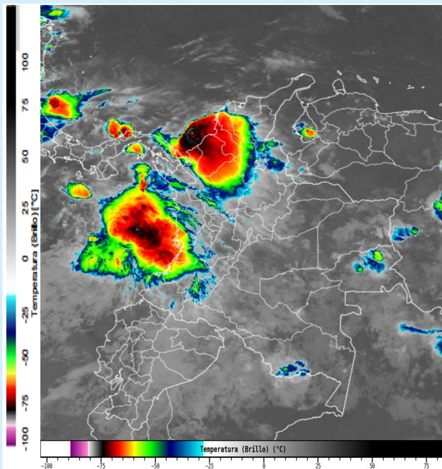
Imagen GOES 19 (East) Canal Infrarrojo 10 de julio de 2025 - Hora 05:10 HLC Fuente: IDEAM
